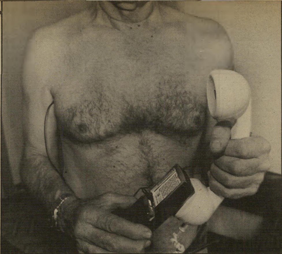
קריאת אזעקה האדם מחובר למכשיר הקרדיוביפר באמצעות שתי אלקטרודות. הקרדיוביפר מוצמד לפומית-הטלפון, ולחיצה על כפתור המכשיר משדרת סידרת ציפופים, הנקלטים דרך מכשיר הטלפון במוקד שח"ל, ומפוענחים באמצעות מחשב לתרשים אק"ג.
